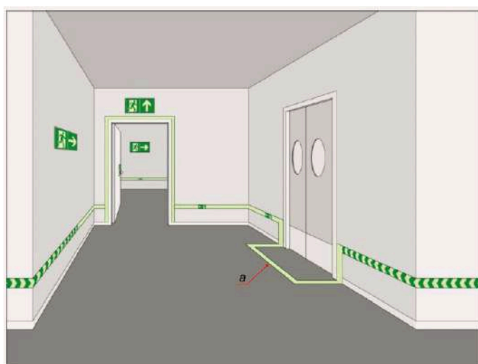
Рисунок В.9 - Пример обозначения тупиков на путях эвакуации в коридорах, проходных помещениях и т.п.
