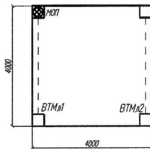
г) ИП линейные дымовые (ВТМл 1-2)
