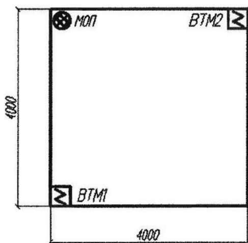
а) дымовые ИП (BTM 1-2)
