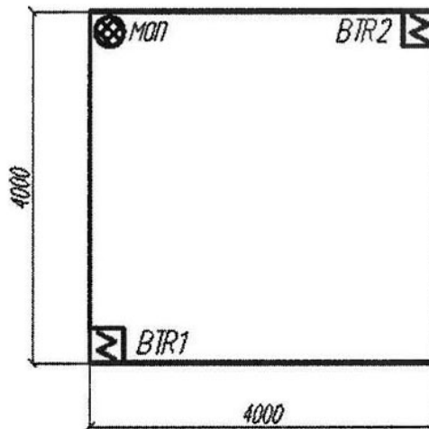
б) газовые ИП (ВТР 1-2)
