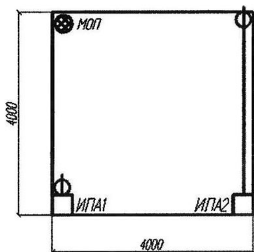
в) аспирационные ИП (ИПА 1-2)
